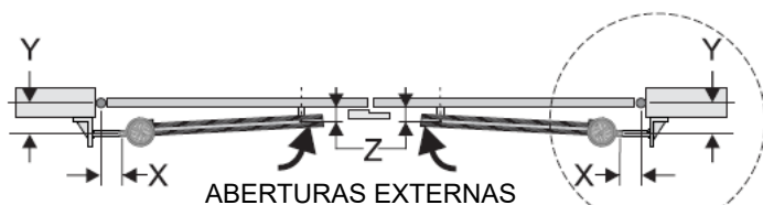
ABERTURAS EXTERNAS
