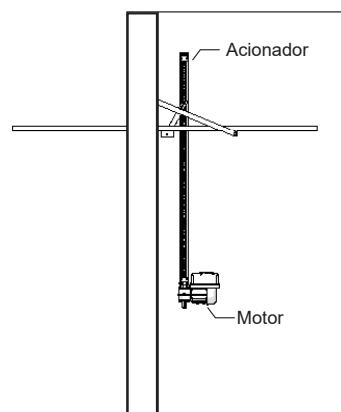
Vista lateral
