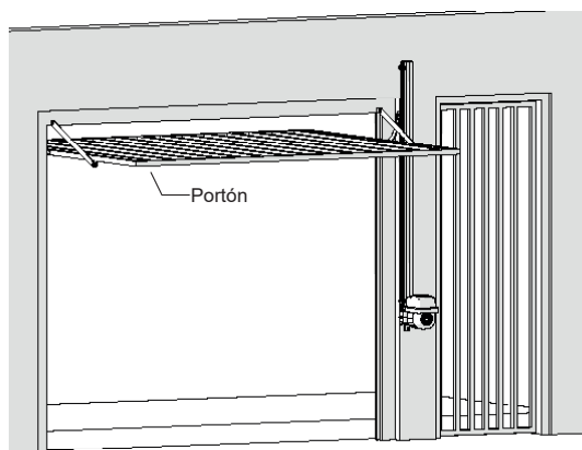
Vista perspectiva
